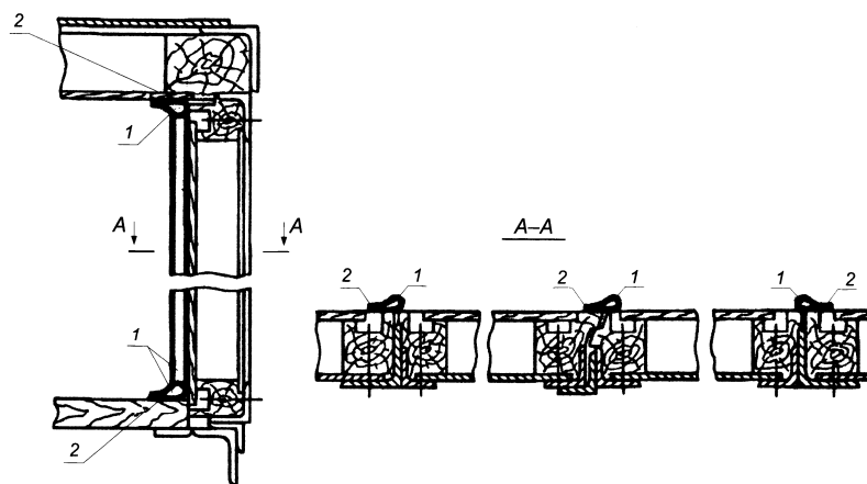
Рис. 8.9. Заделка щелей бумагой в дверном проеме контейнера:
